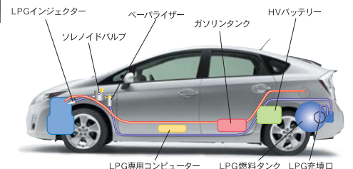
RHYBRID<構造図> — ガソリン燃料配管 — LPG燃料配管
